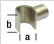
107.308 Siebreflektor, aufziehbar (a x b) 50 x 34 mm 107.309 35 x 20 mm
